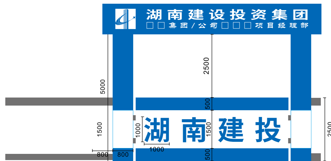
门楼式大门
